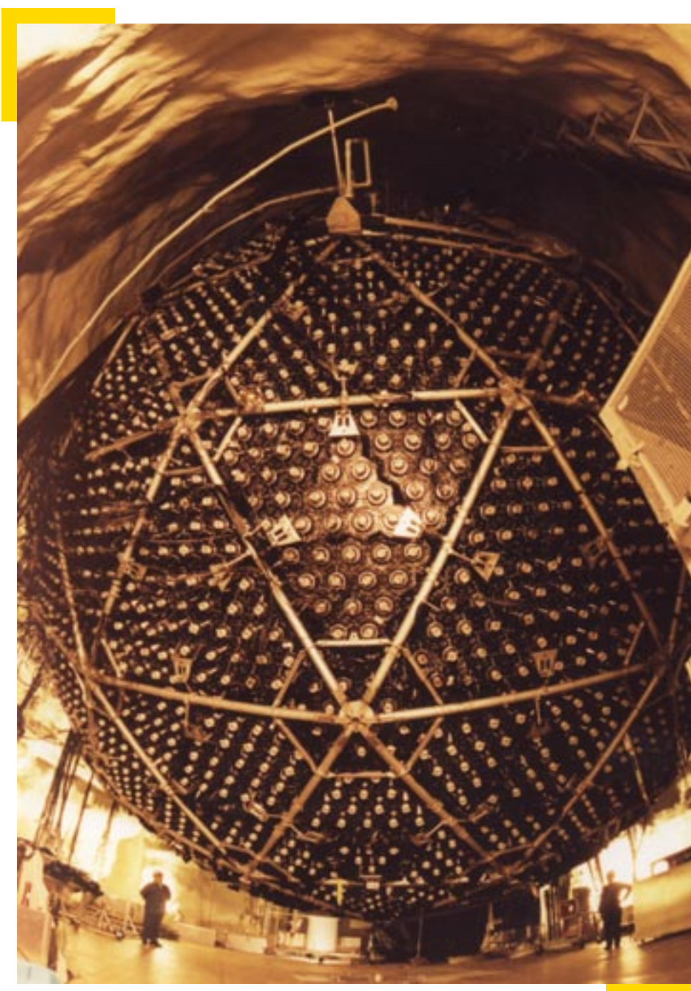
Le détecteur SNO, situé à plus de 2000 mètres de profondeur dans une mine canadienne, est un réservoir de 1000 tonnes d'eau lourde, capable de détecter et d'identifier les neutrinos.
