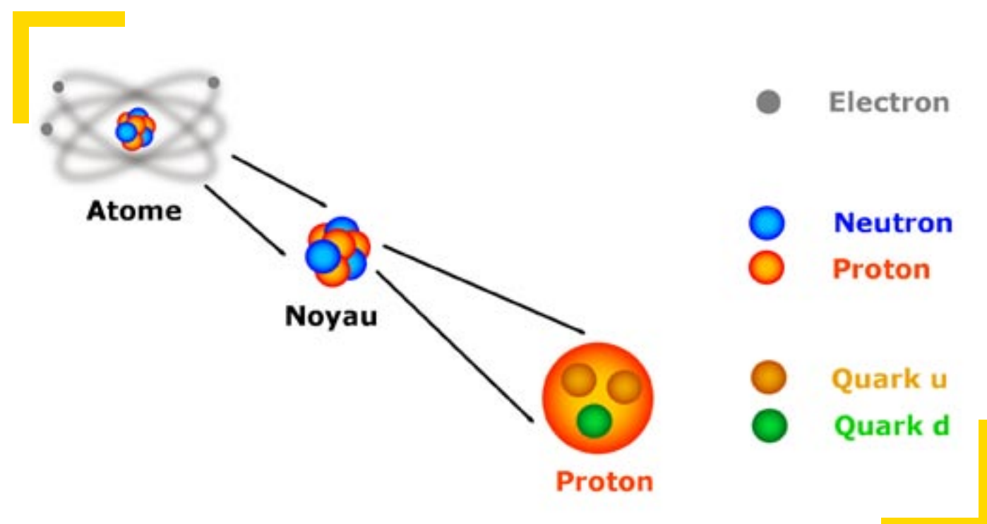
Les constituants de la matière, depuis l'atome jusqu'au quark.
