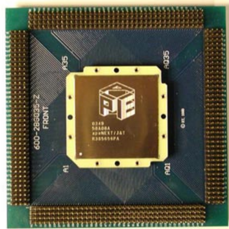
Une puce de l'ordinateur apeNEXT, conçu en partie au LPT. Cette machine a été spécialement créée pour effectuer des simulations sur ordinateur de l'interaction nucléaire forte qui lie les quarks entre eux dans les protons et les neutrons.
